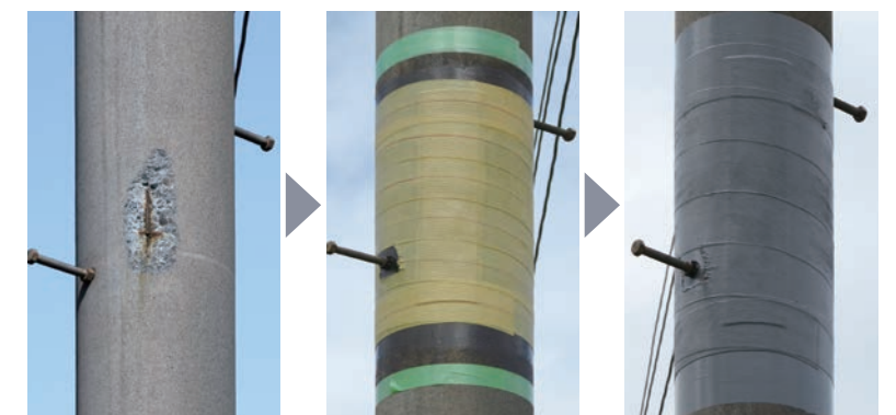
補修前 アラミド補修状況 補修完了
